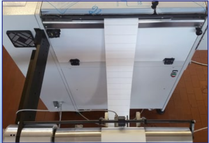
Opzione syncro in linea/ on line syncro kit
